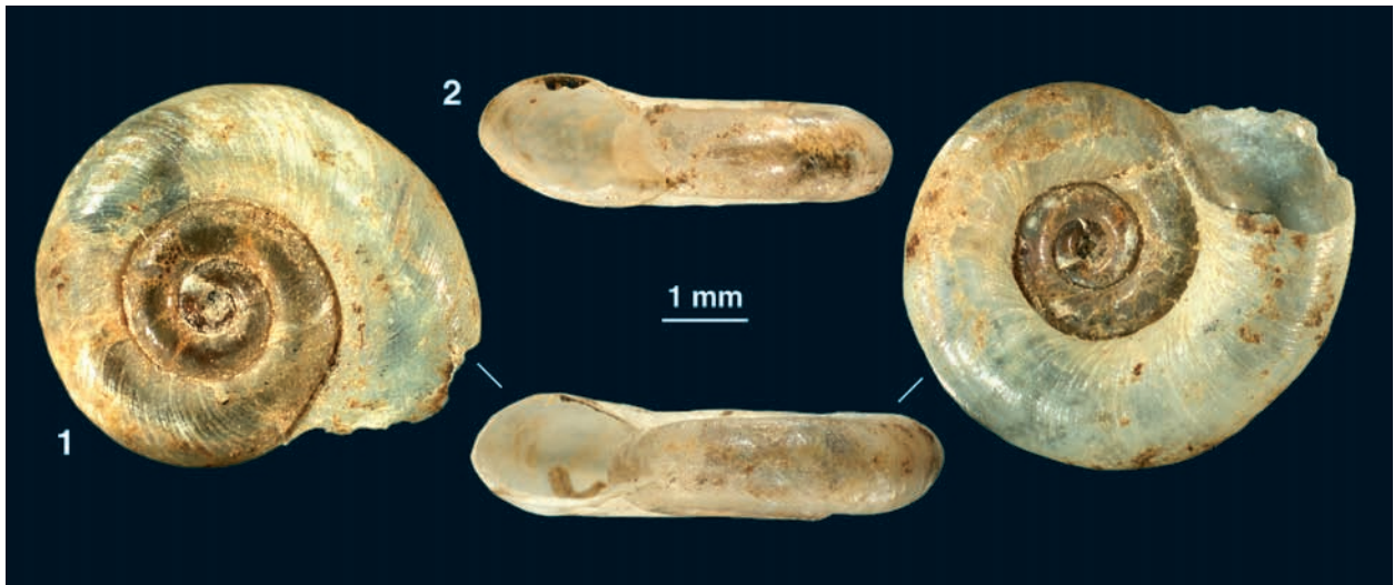
Abb. 5. Gyraulus hebraicus , 1: Paralectotypus, 2: Lectotypus.
